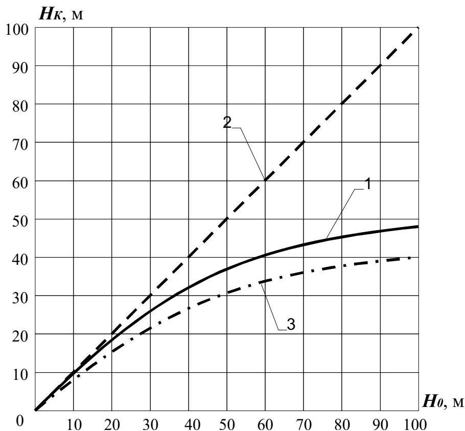
Рисунок 2 – Залежність H_k від H_0 для круглого струменя з лафетного ствола з d_H = 25 мм: 1 – фактичні дані; 2 – з урахуванням тільки сил поверхневого натягу; 3 – з урахуванням тільки сил в'язкості [3; 4].
