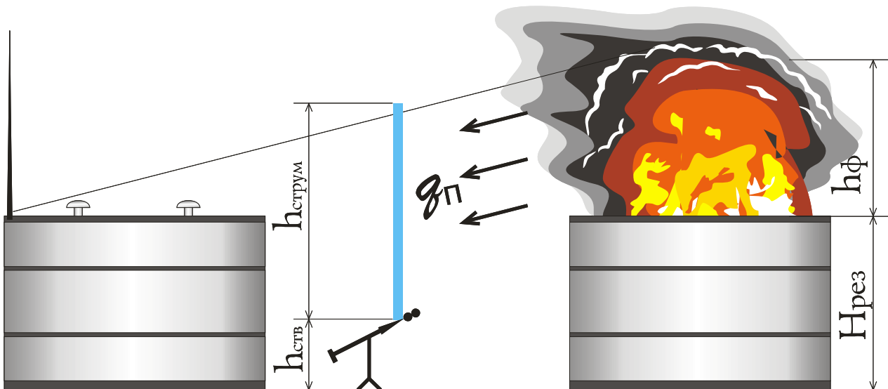
Рисунок 3 – Принципова схема захисту резервуара з нафтопродуктом від теплового потоку факела полум'я за допомогою водяної завіси-екрана.
